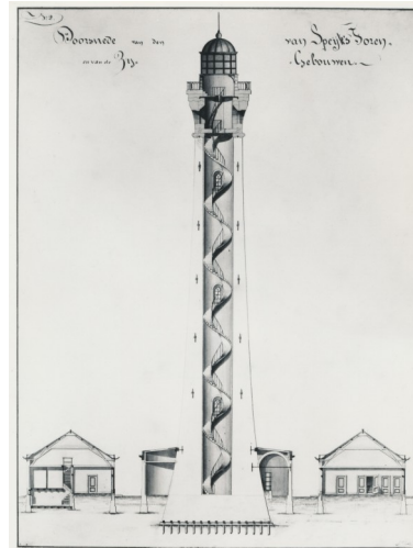
Ontwerp voor de Van Speyk kustlichtto- ren uit 1833. De toren bestaat uit slechts één cilinder.
