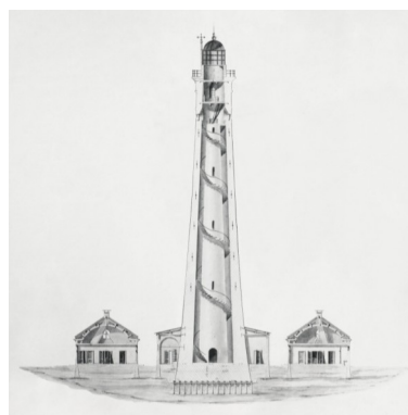
De vuurtoren van West-Schouwen in 1840. De toren bestaat uit twee cilin- ders, met daartussen een wenteltrap.
